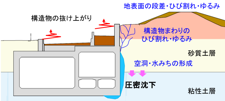
地盤変形(不同沈下)による被害想定
