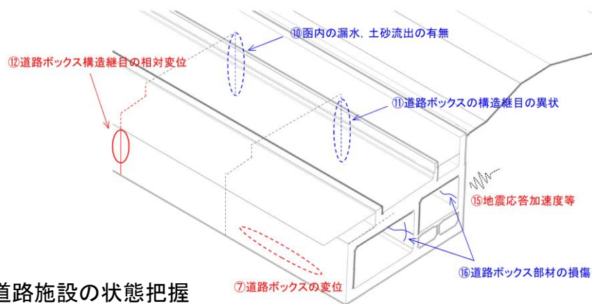
(a) 河川堤防の状態把握
