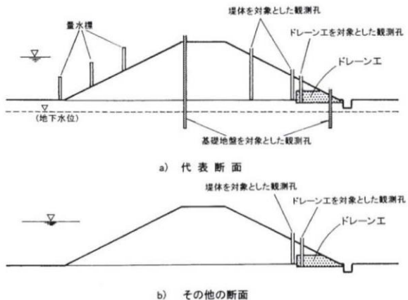
観測施設の標準的な配置 (ドレーン工設計・施工に関する参考資料(技術資料)より引用)
