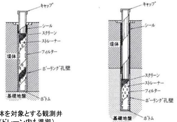
基礎地盤を対象とする観測井 (ドレーン工設計・施工に関する参考資料(技術資料)より引用)
