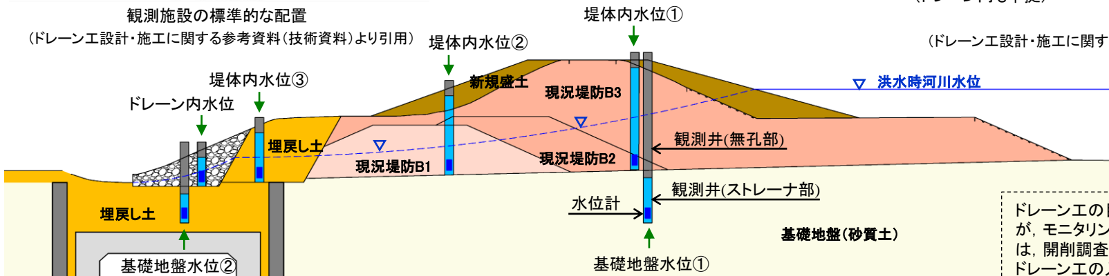
堤体を対象とする観測井 (ドレーン内も準拠)
