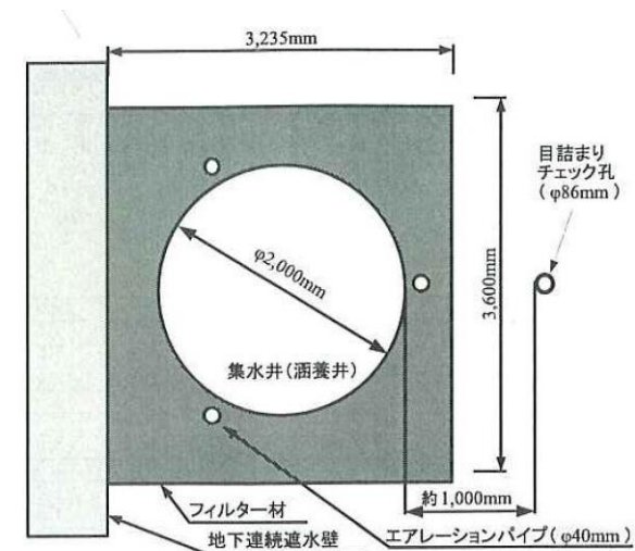
【阪和自動車道堺地区工事での対策事例】
