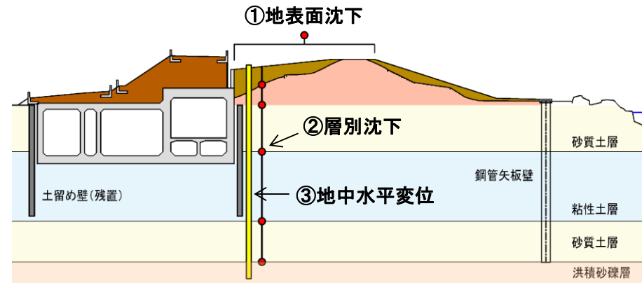
地盤変位計測モニタリング
