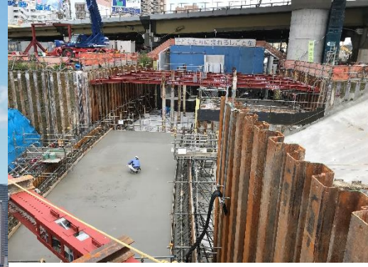
②擁壁部の躯体工
