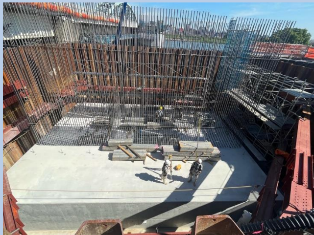
①橋脚基礎のコンクリート打設
