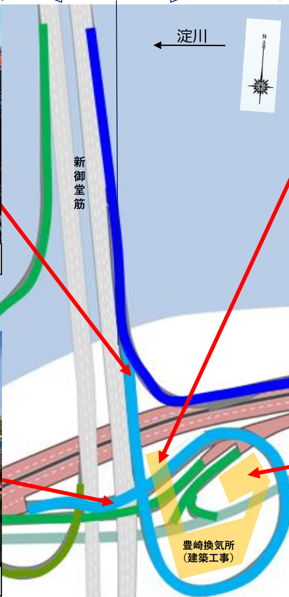
③擁壁部の底版コンクリート打設
