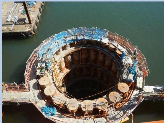
①河川内の 鋼管矢板井筒基礎
