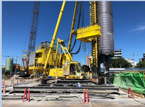
②地中連続壁(土留)施工
