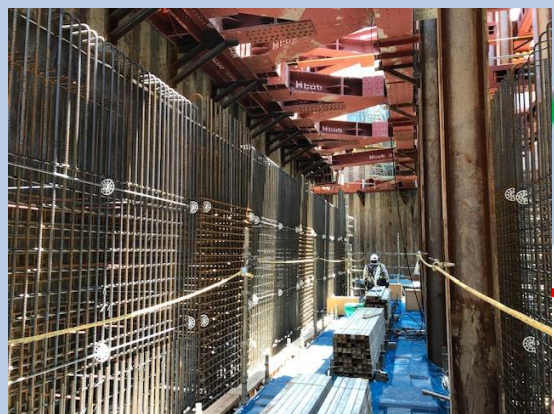
躯体施工
