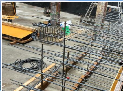
④底版コンクリートの型枠組立
