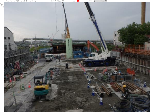
⑥地盤改良
