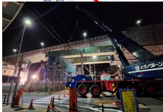
④橋桁の設置
