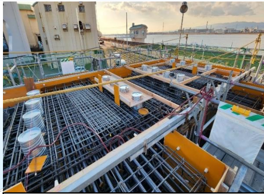
②橋脚本体の構築
