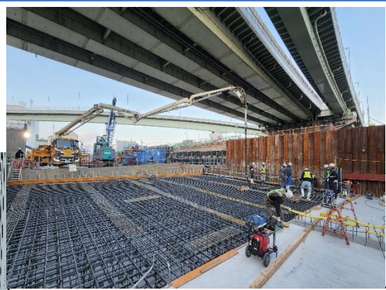
②掘割擁壁部の構築
