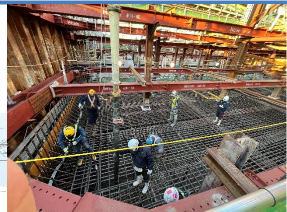
③掘割擁壁部の構築
