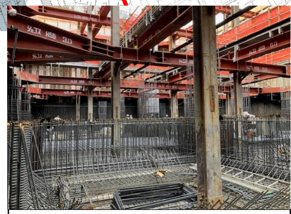
⑤換気所地下部の構築
