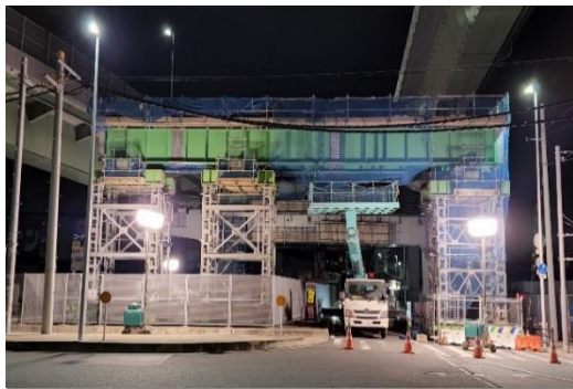
④ベントの設置
