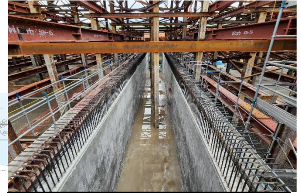
③トンネル本体の構築
