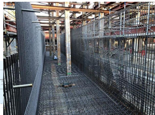
③トンネル本体の構築
