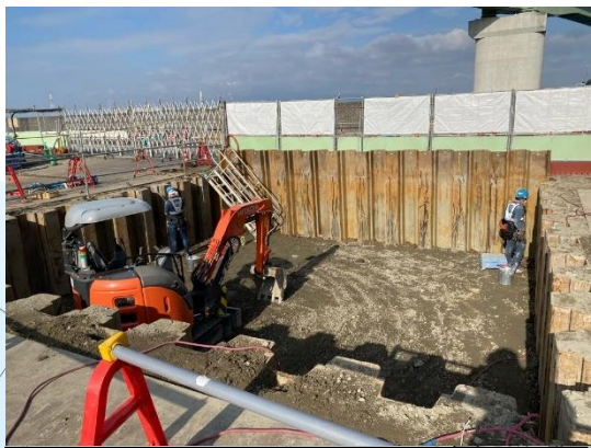
橋台部の掘削
