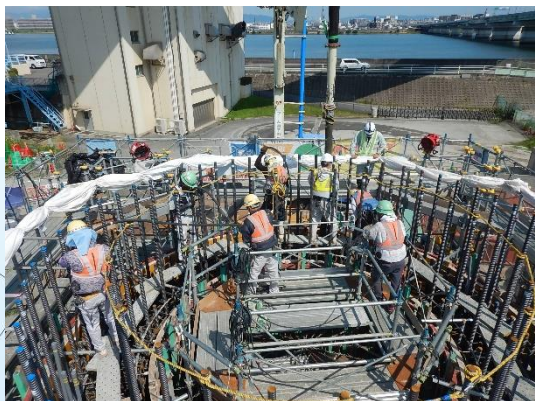
橋梁基礎の構築
