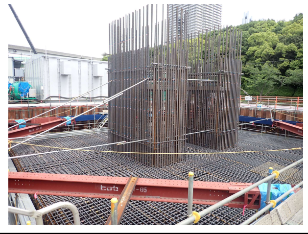
【1】高速道路の橋脚(PE-1)基礎工事に於いて、フーチング・橋脚構築に向けた鉄筋組立中。
