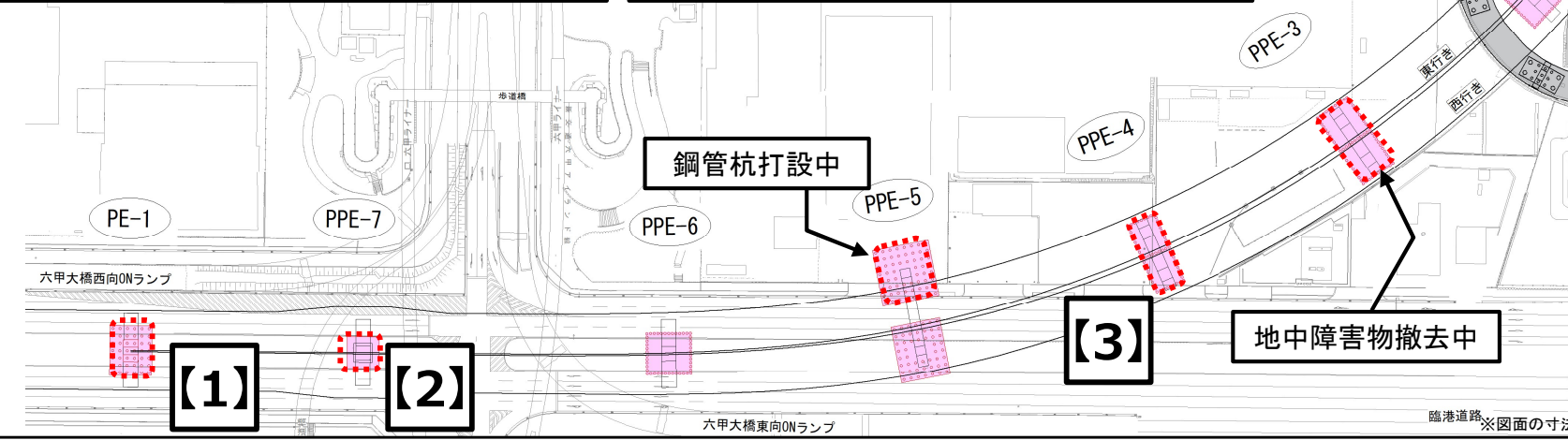
【3】高速道路の橋脚(PPE-4)基礎工事に於いて、鋼管矢板基礎施工前の先行削孔中。
