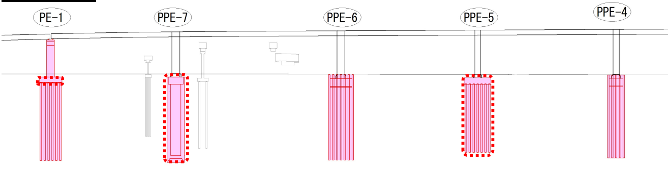
縦断面図 (西行)
