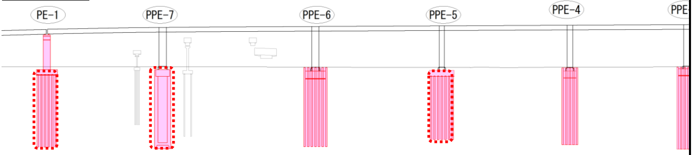
縦断図 (西行)
