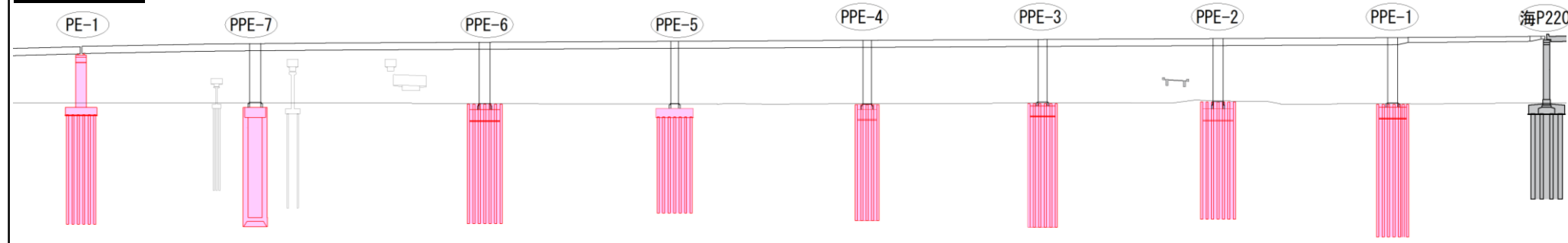
縦断図 (西行)
