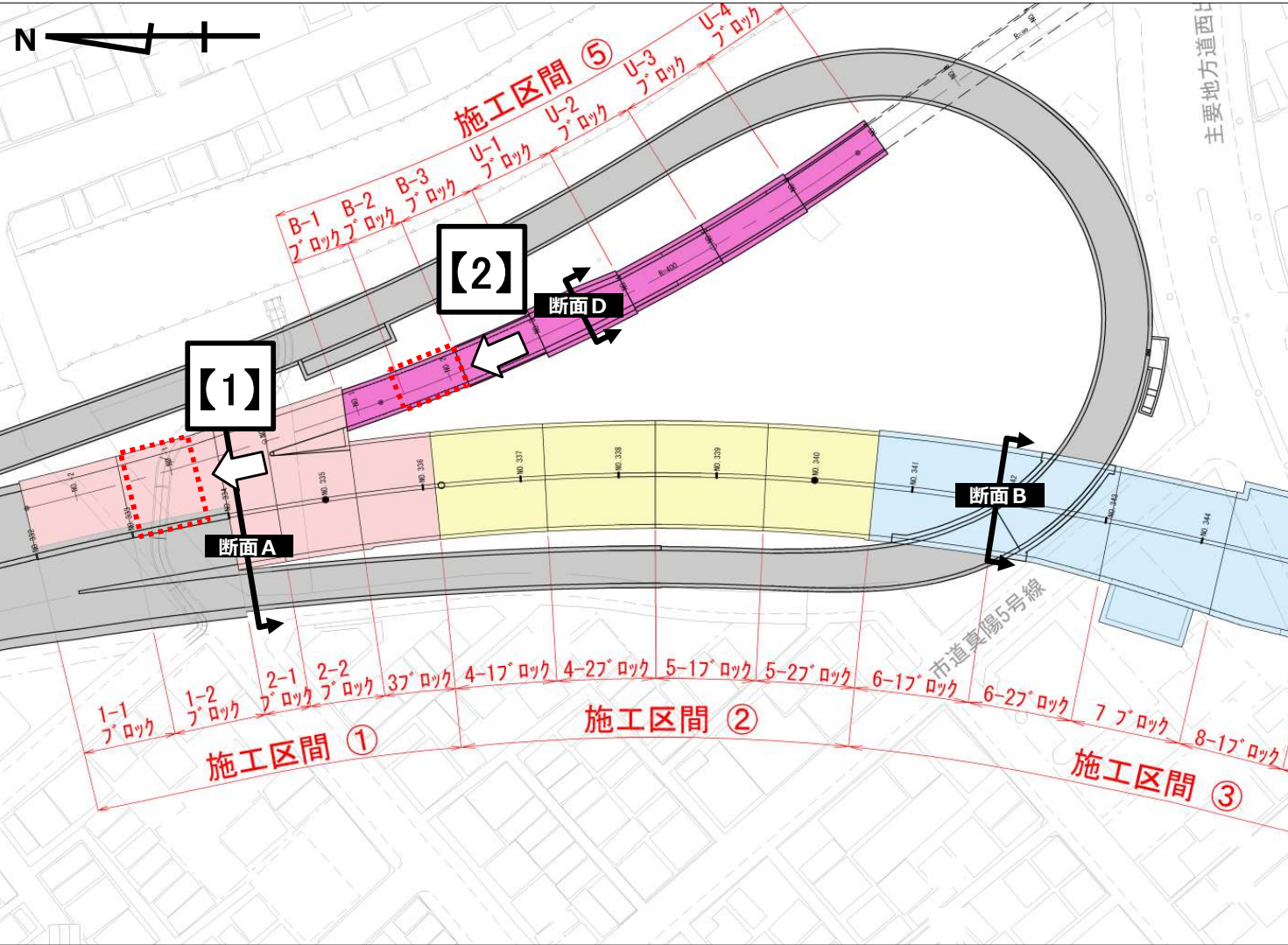
【1】施工区間① 1-2ブロック 掘削状況
