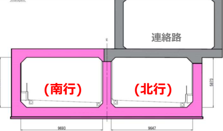
断面 B
