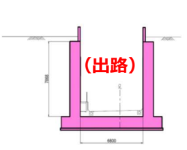
断面 D
