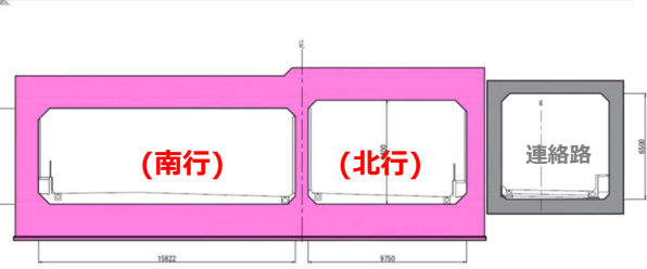
断面 A
