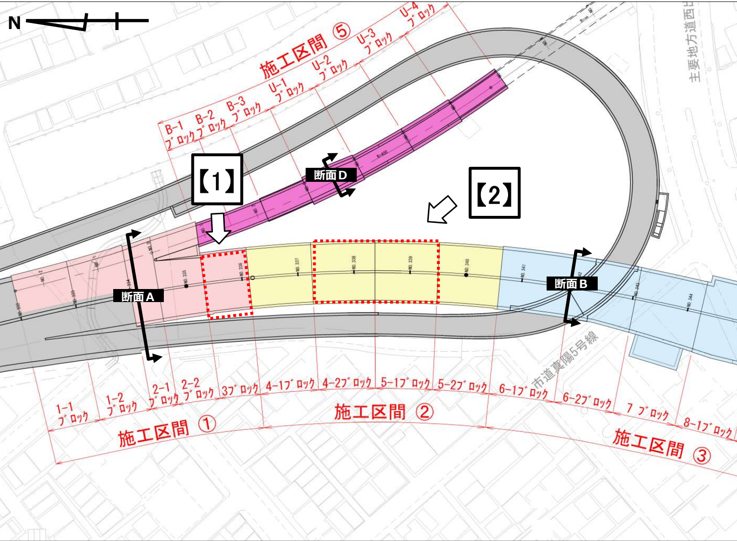
【1】施工区間① 3ブロック 掘削状況
