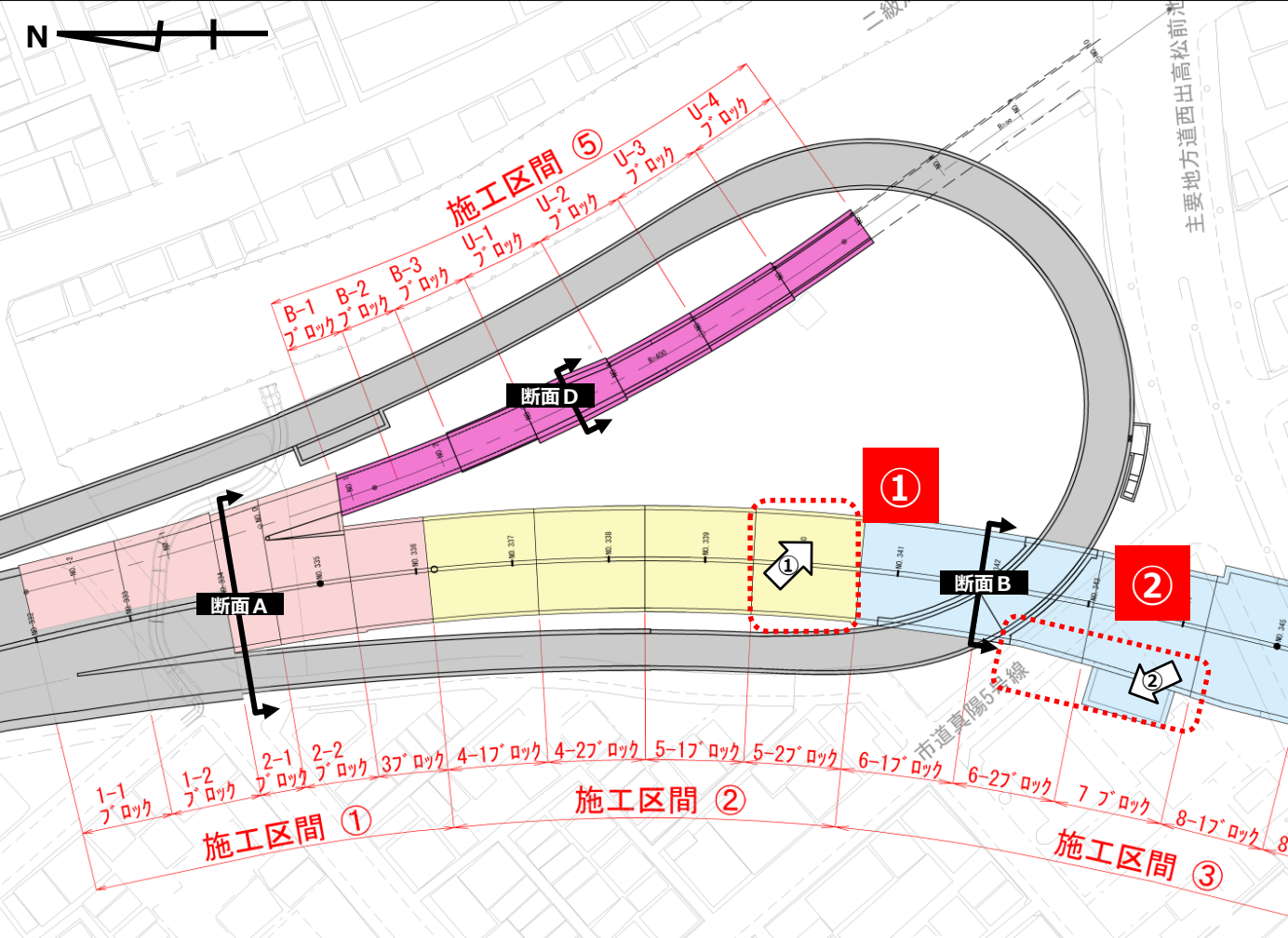
①頂版部の型枠、鉄筋組立が完了したため、頂版コンクリート打設を実施。
