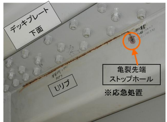
鋼床版のデッキプレートとウリブ溶接部のき裂
